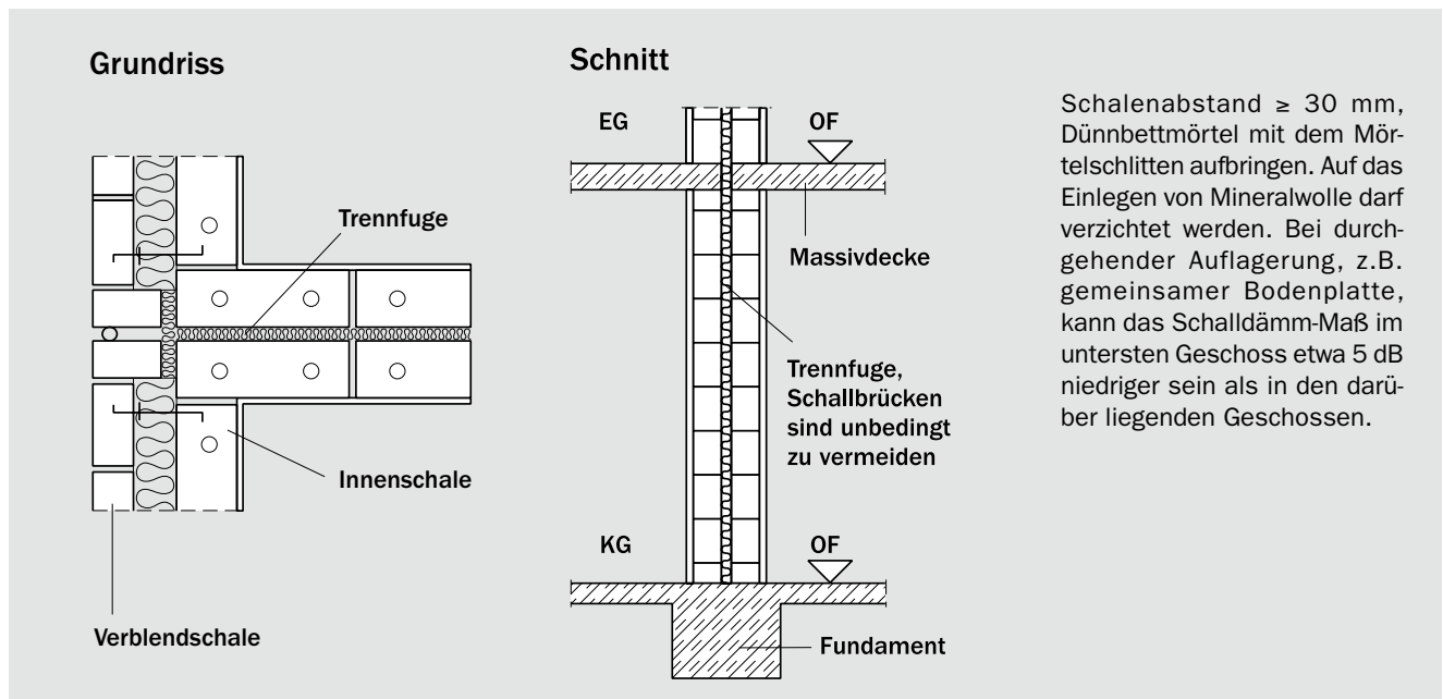
Bild 4: Ausführungsbeispiel für zweischalige Trennwand aus zwei schweren, biegesteifen Schalen mit bis zum Fundament durchgehender Trennfuge.
