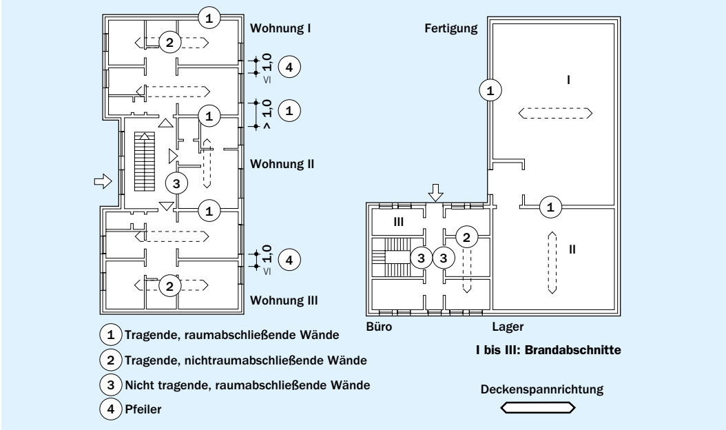
Bild 1/1 Brandschutztechnische Klassifizierung von Wänden im Wohn- und Industriebau
