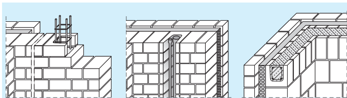
Aussteifungsstütze mit KS-U-Schalen
